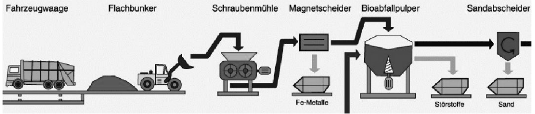
Grafik, Funktionsschema der Vergärungsanlage in Kirchstockach, Auszug, Störstoffbeseitigung Quelle Landratsamt München
